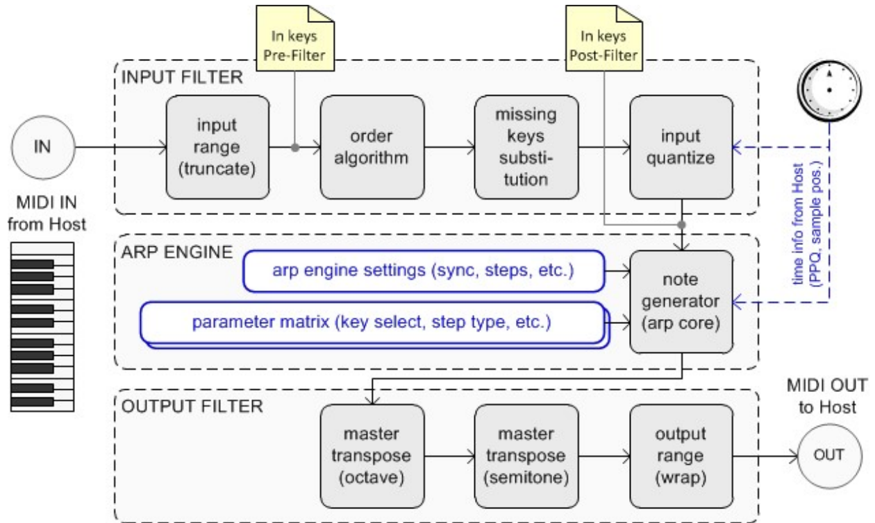
pic. 1. BlueARP: Блок-схема.
